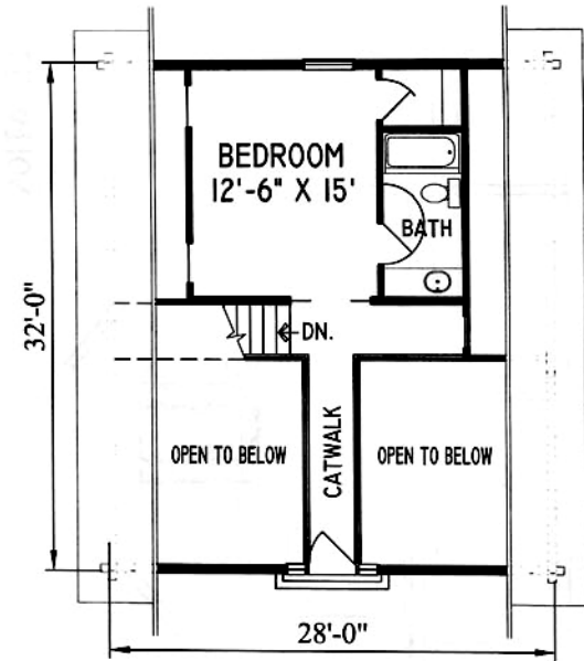
LOFT PLAN
